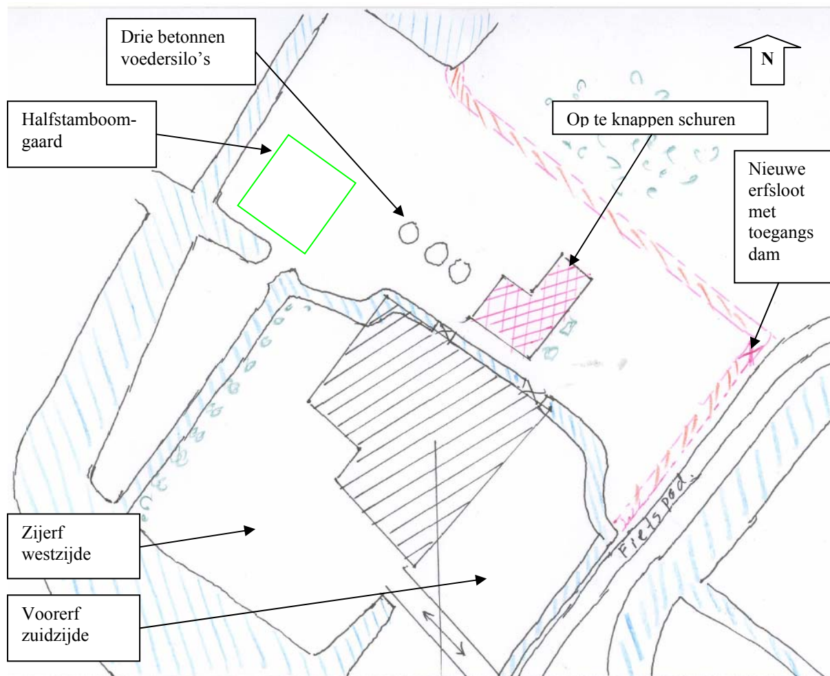
Figuur 3. Situatietekening Holyweg 16 (tekening van Aad Kleyweg op basis kadastrale gegevens). Rood gearceerd: de nieuwe erfsloot.
